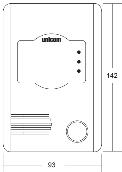
【外型尺寸】
