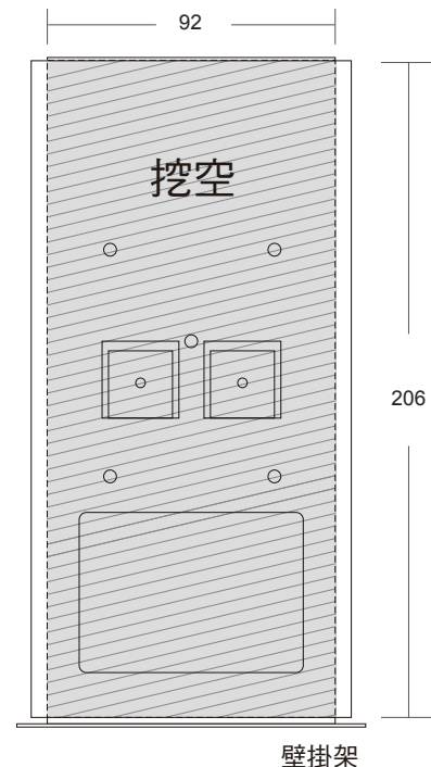
【開孔尺寸】
