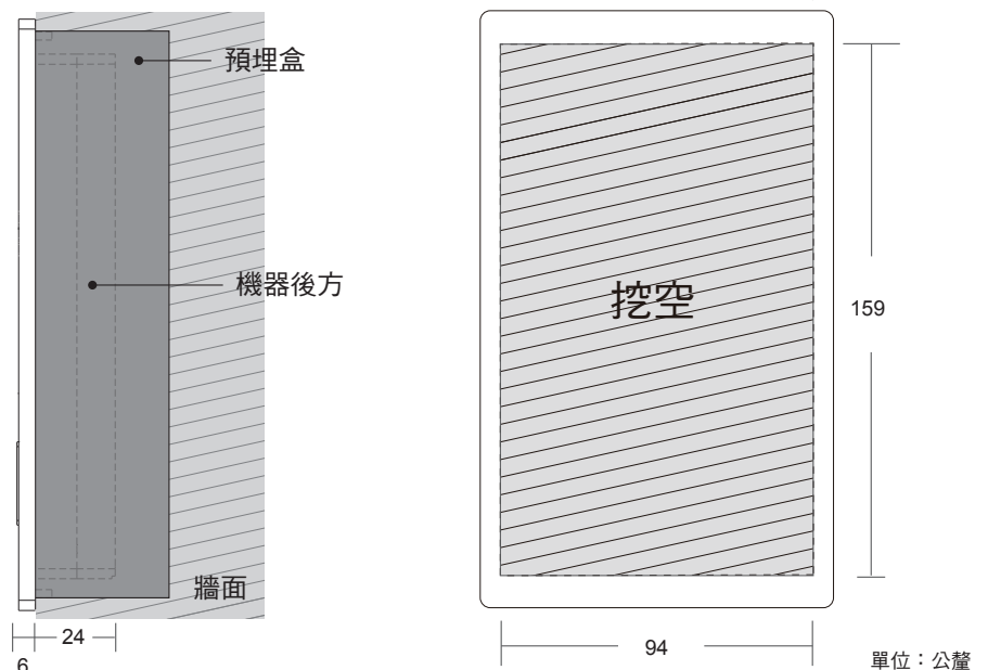
【開孔尺寸】
